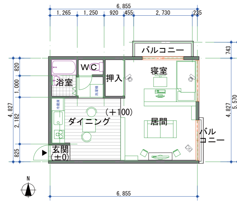
平面図 S1/100
