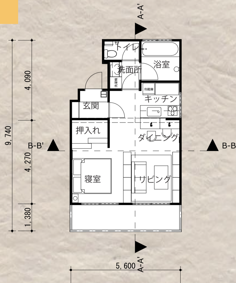
平面図
